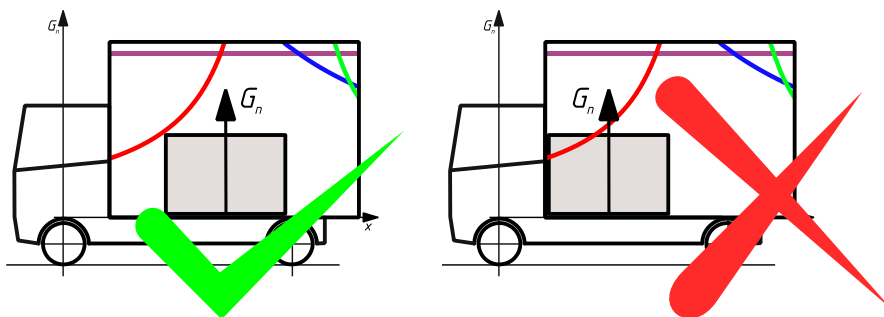
Slika 32: Pravilna in napačna namestitvev tovora glede na porazdelitveni diagram
