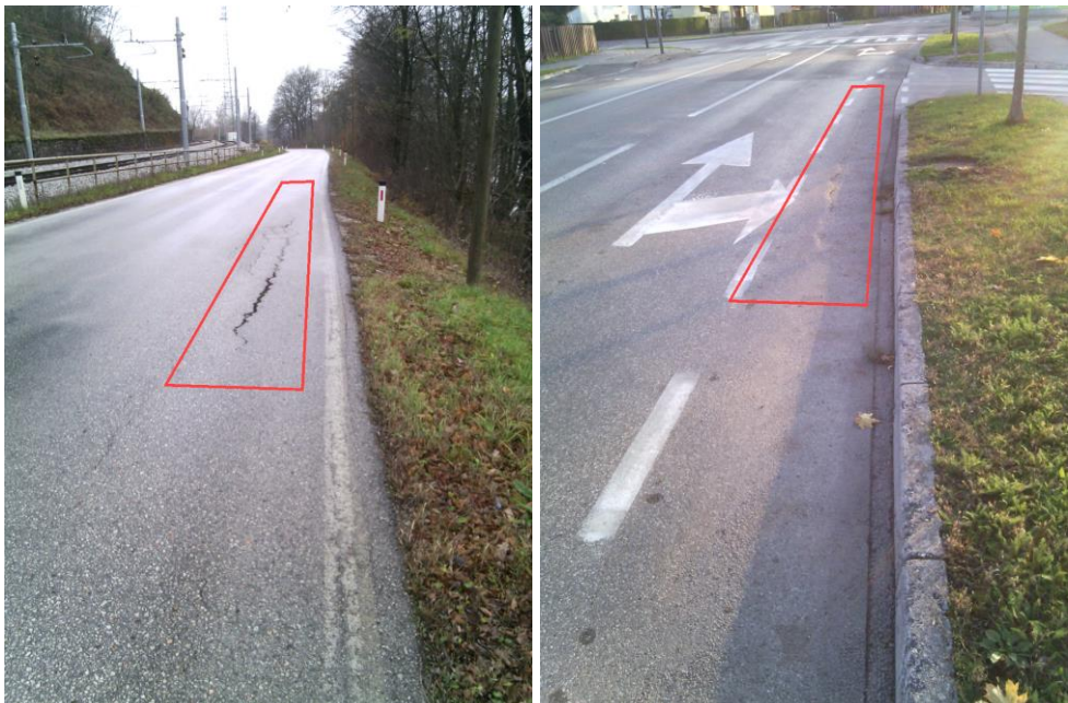
Slika 78: Poškodbe vozišča zaradi pretežkih vozil (levo razpoka, desno vdolbina)
