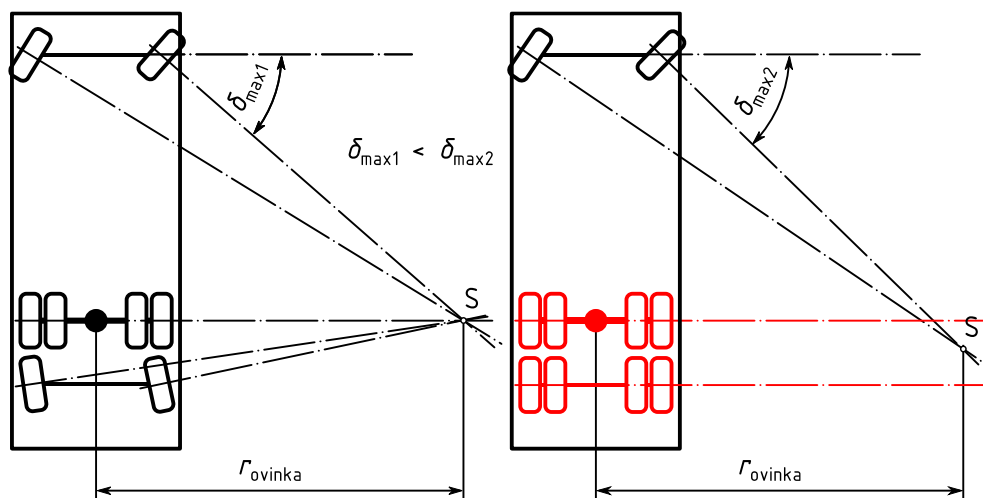
Slika 57: Geometrija krmiljenja trisosnega vozila
