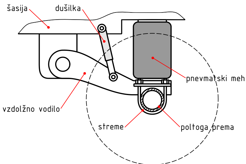
Slika 51: Pnevmsko vzmetenje poltoga preme
