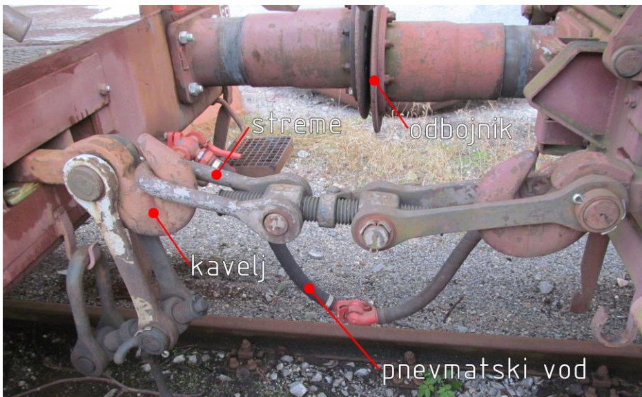
Slika 129: Tovorna vagona speta z vijačno spenjačo
